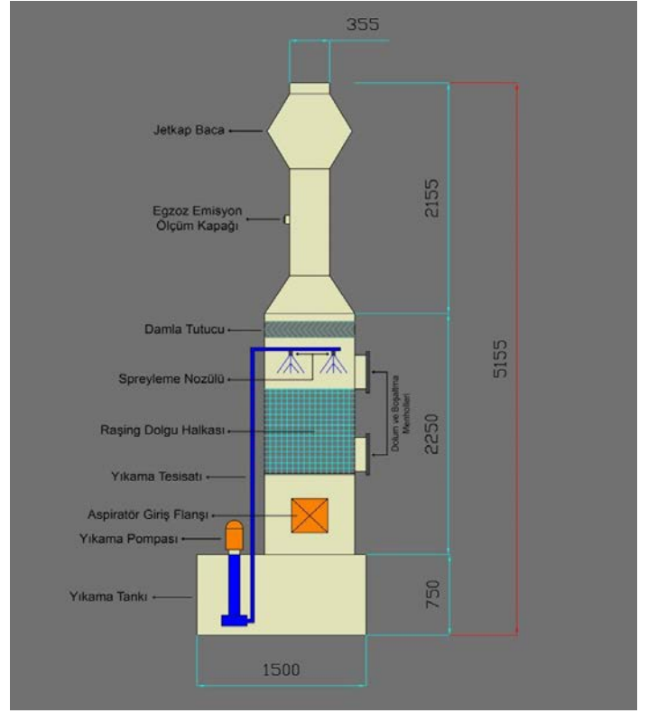
SCRUBER TEKNİK ÇİZİMİ
